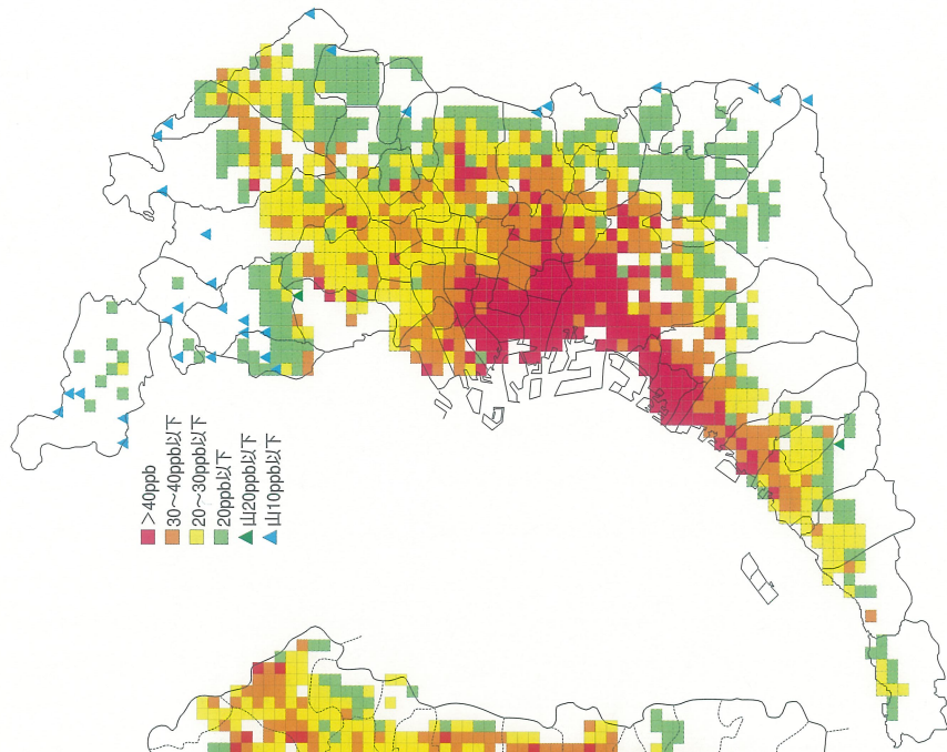
2006年NO 2 測定濃度分布図 (2006年5月18日18:00~19日18:00)
