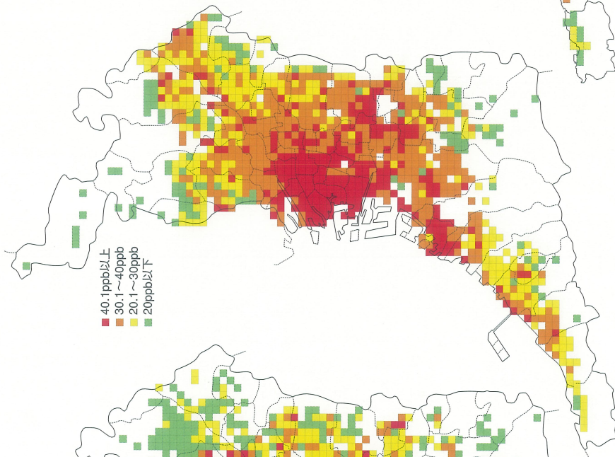
2000年度NO 2 測定濃度分布図 (2000年5月18日18:00~19日18:00)
